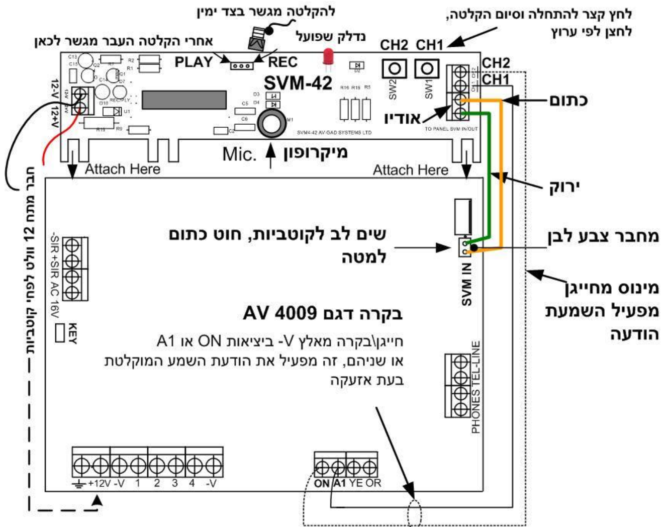
איור 1: תאור חבורים וחיווט מודול הקלטה לבקרה 4009
