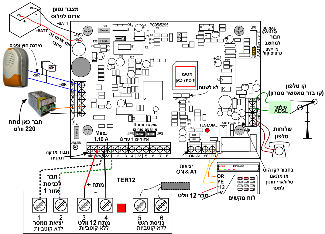
איור 3: חבר תרמוסטט - לבקר חייגן אב-גד
